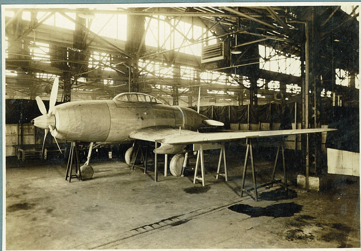
寫 眞 1 全 体
