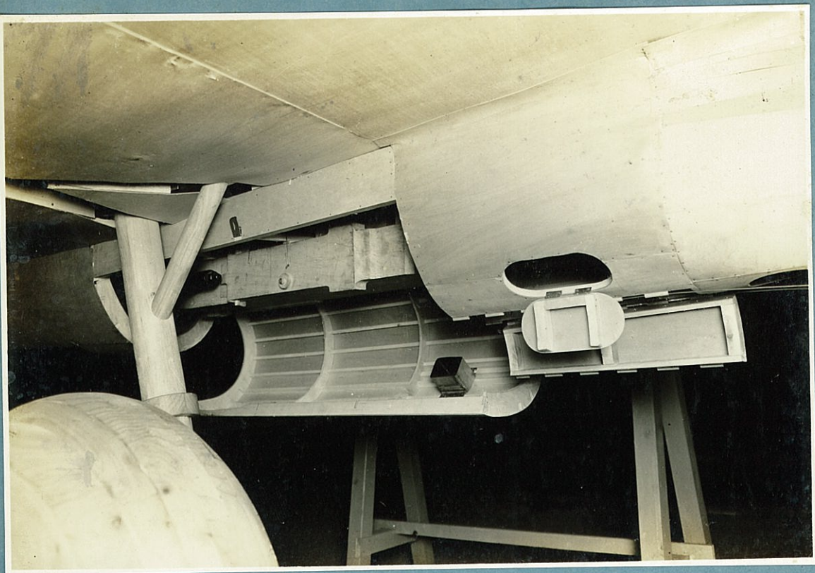
寫真 5 砲取付（其ノ一）
