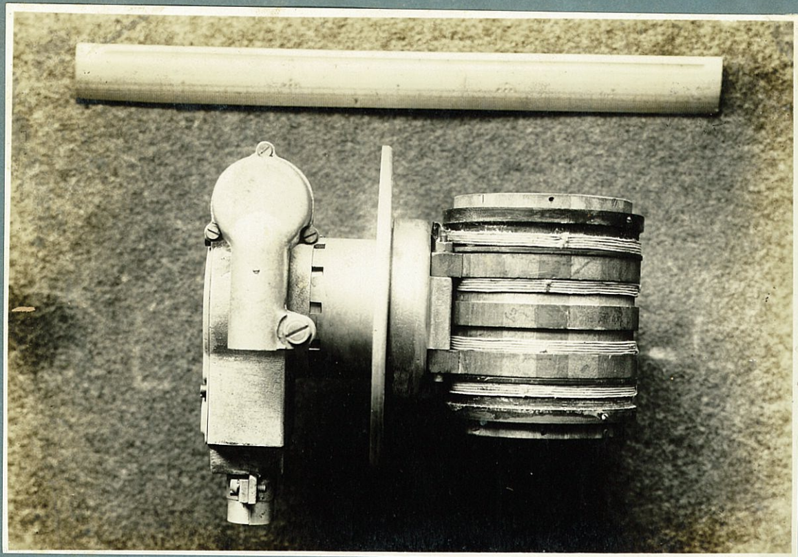
寫・眞 17 方向探知器 (其ノ三)
