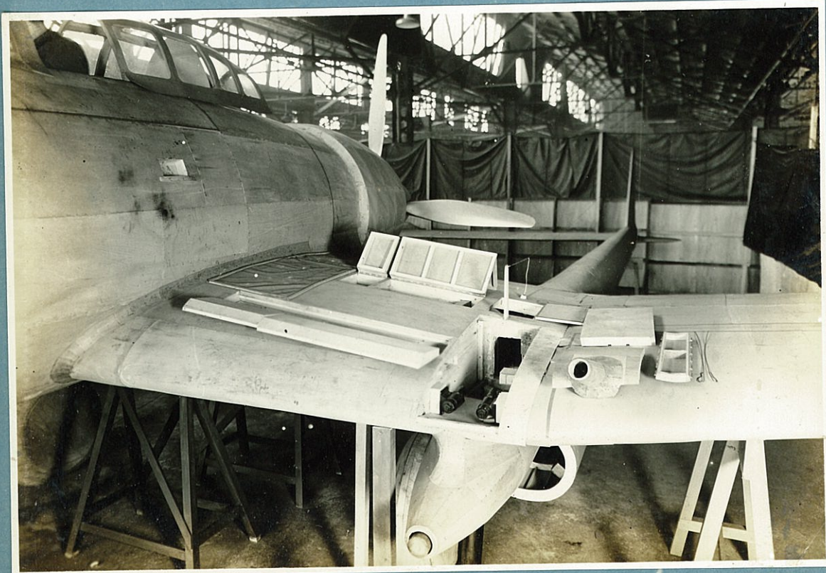
寫真 6 砲取付（其ノ二）
