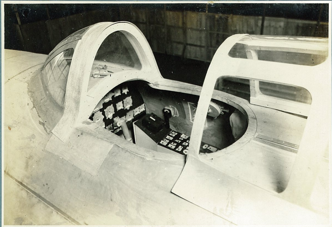
寫真 7 操縱席
