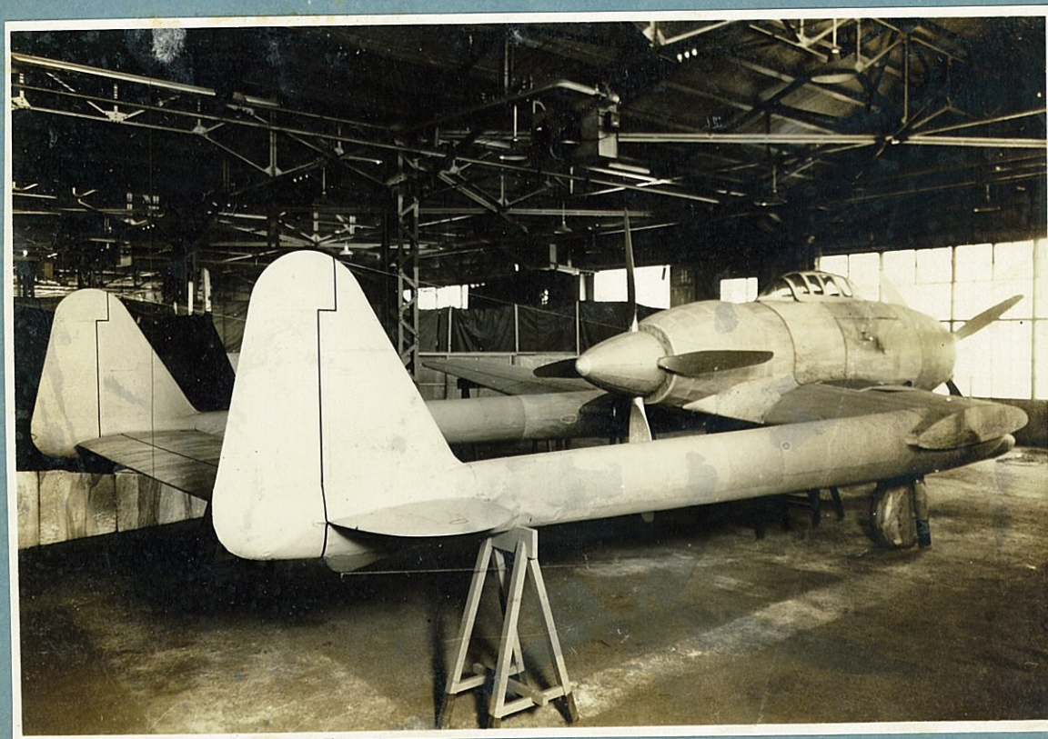
寫 眞 2 斜 後 面
