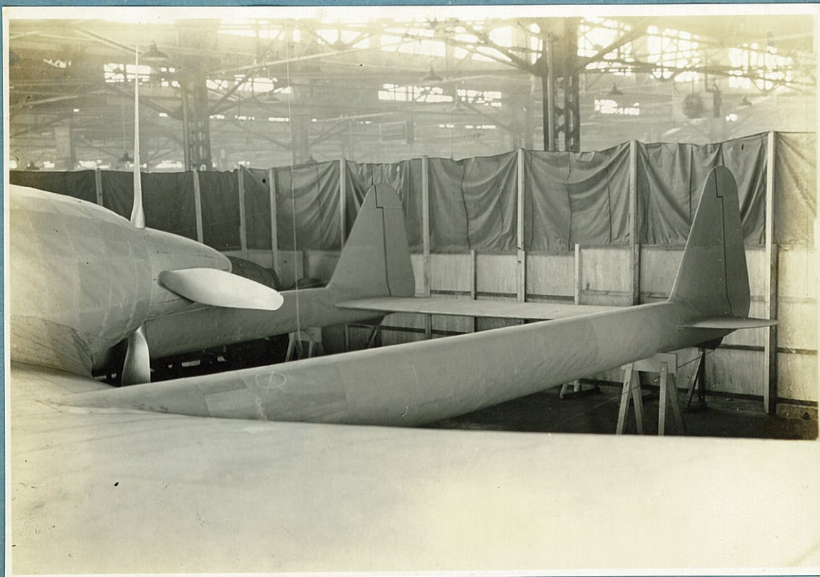
寫真 4 支 柱
