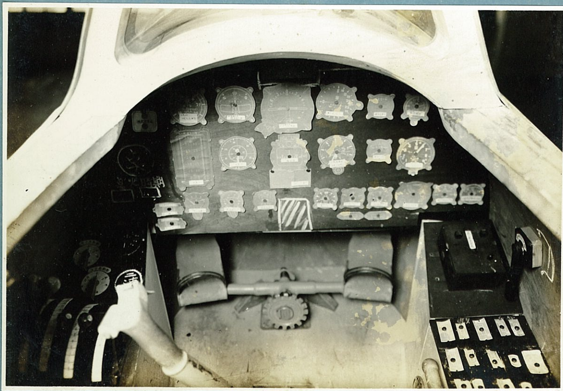
寫真 10 計器板
